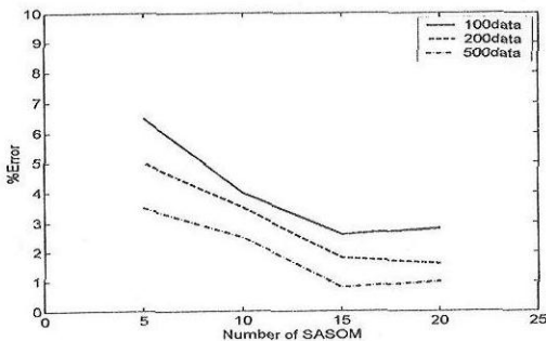
그림 4. 양상블의 에러율
