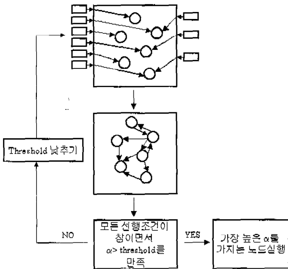
그림 7 행동 네트워크의 행동선택 과정( \alpha = 활성화도값)
